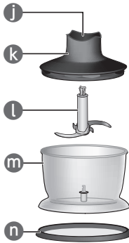
チョッパー
